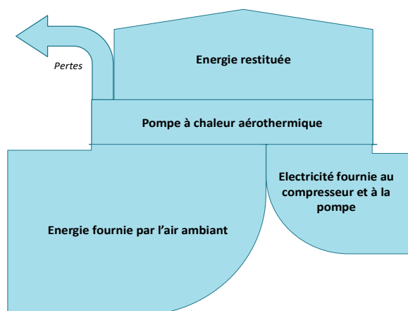
Figure 39 : Flux d'énergie simplifié pour les PAC aérothermiques
