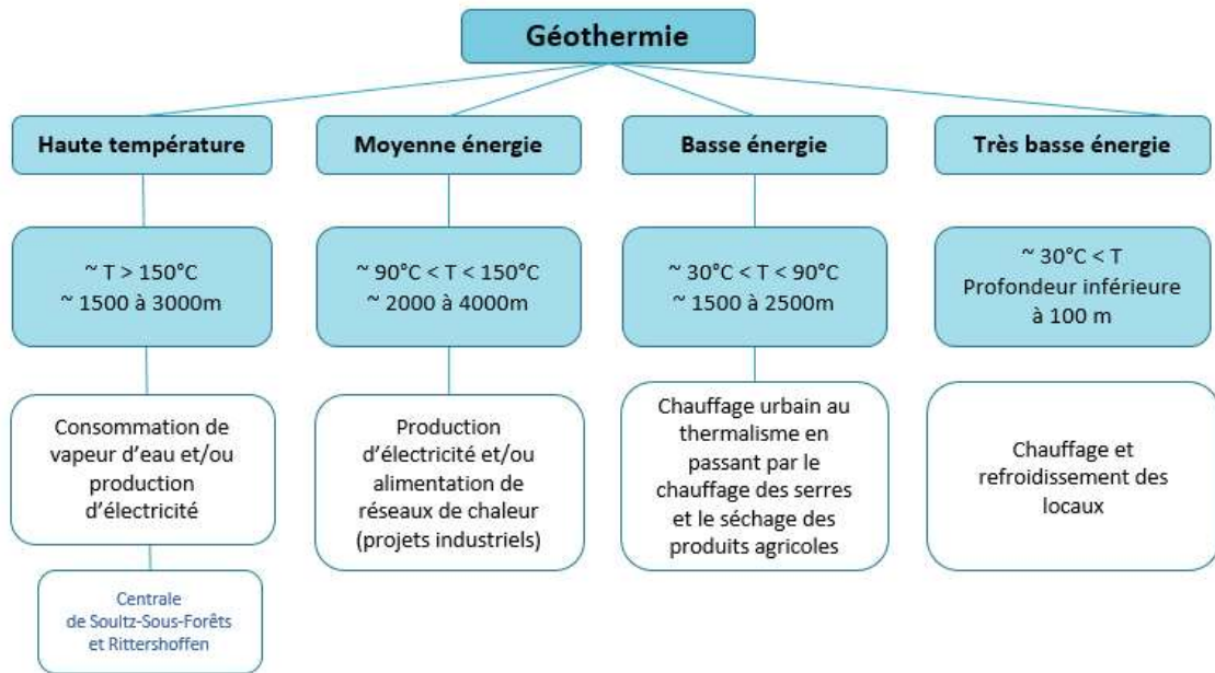
Figure 35 : Géothermie haute, moyenne, basse et très basse énergie : températures, profondeurs, mode d'exploitation et applications : schéma réalisé à partir des descriptions d'Observ'ER.
