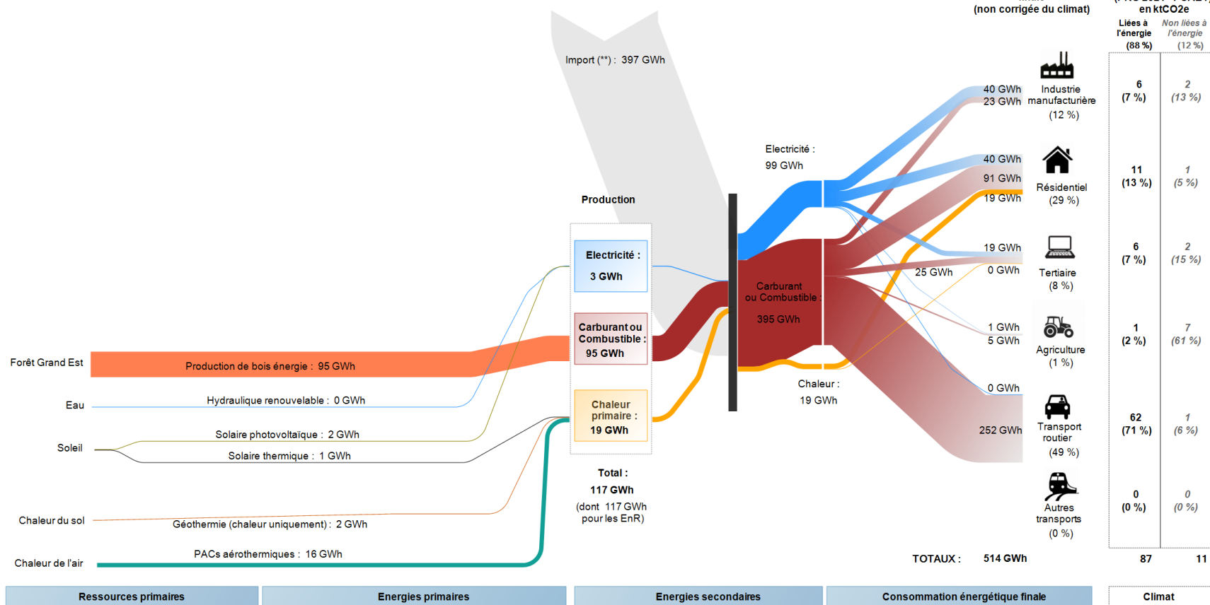
Diagramme de flux des productions d'énergie primaire et des consommations énergétiques finales en 2022 PTRTE de la CC de la Vallée de la Doller et du Soultzbach
